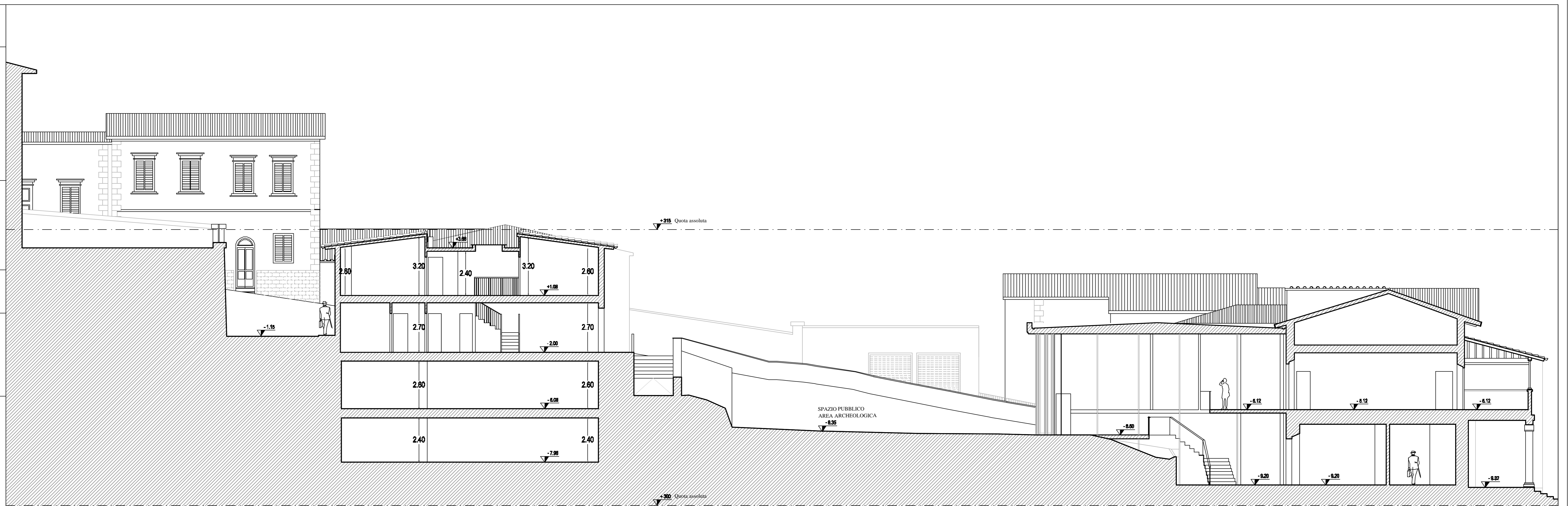
Sezione GG
