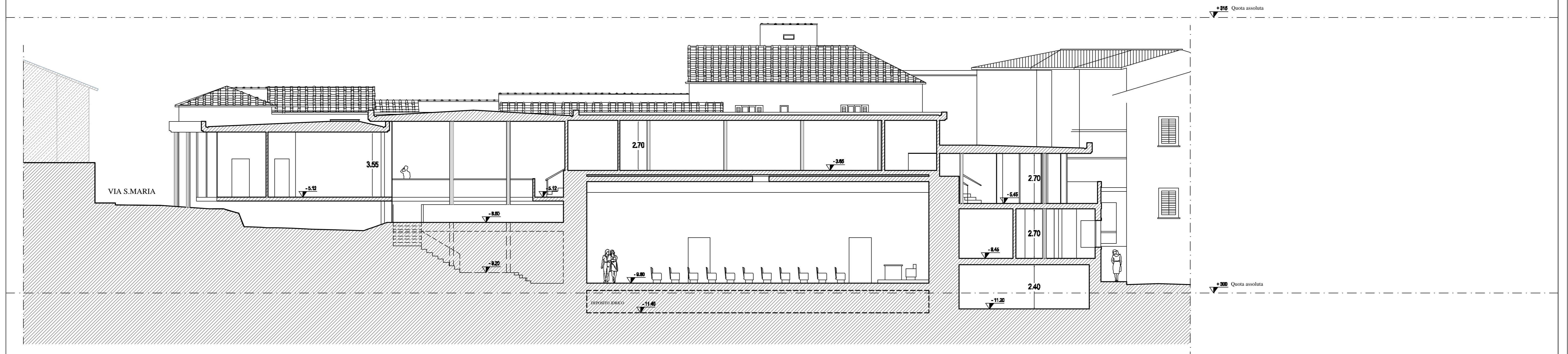
Sezione HH
